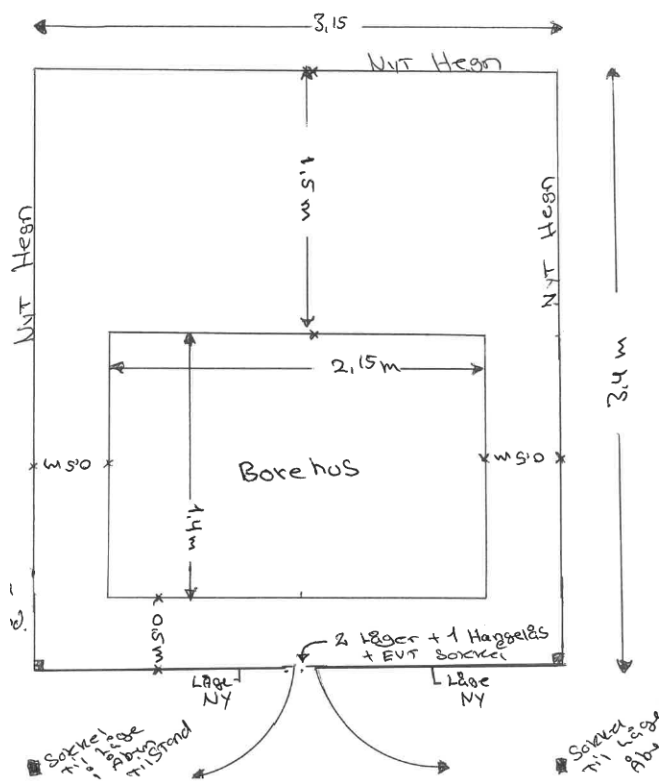
Figur 2 Skitse til mål og design af raftehegn omkring borehuse
